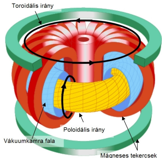
1. ábra: Tokamak vázlatos felépítése és a toroidális geometria irányai
